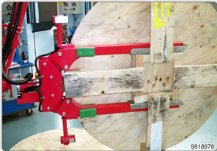
Приспособление для захвата и ручного поворота специальных поддонов.
