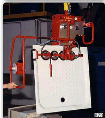
Манипулятор с приспособлением с присосами ("Venturi") для захвата и перемещения душевых поддонов.
