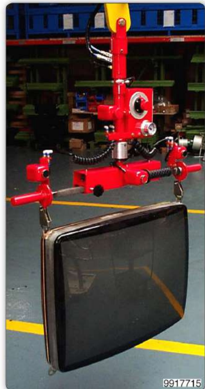
Манипулятор с крюковым приспособлением с регулируемым межкрюковым расстоянием между крюками для перемещения кинескопа с захватом за суппорт.
