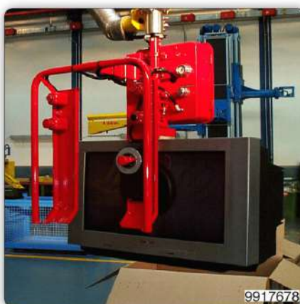
Манипулятор с приспособлением с присосами для захвата и перемещения телевизоров.
